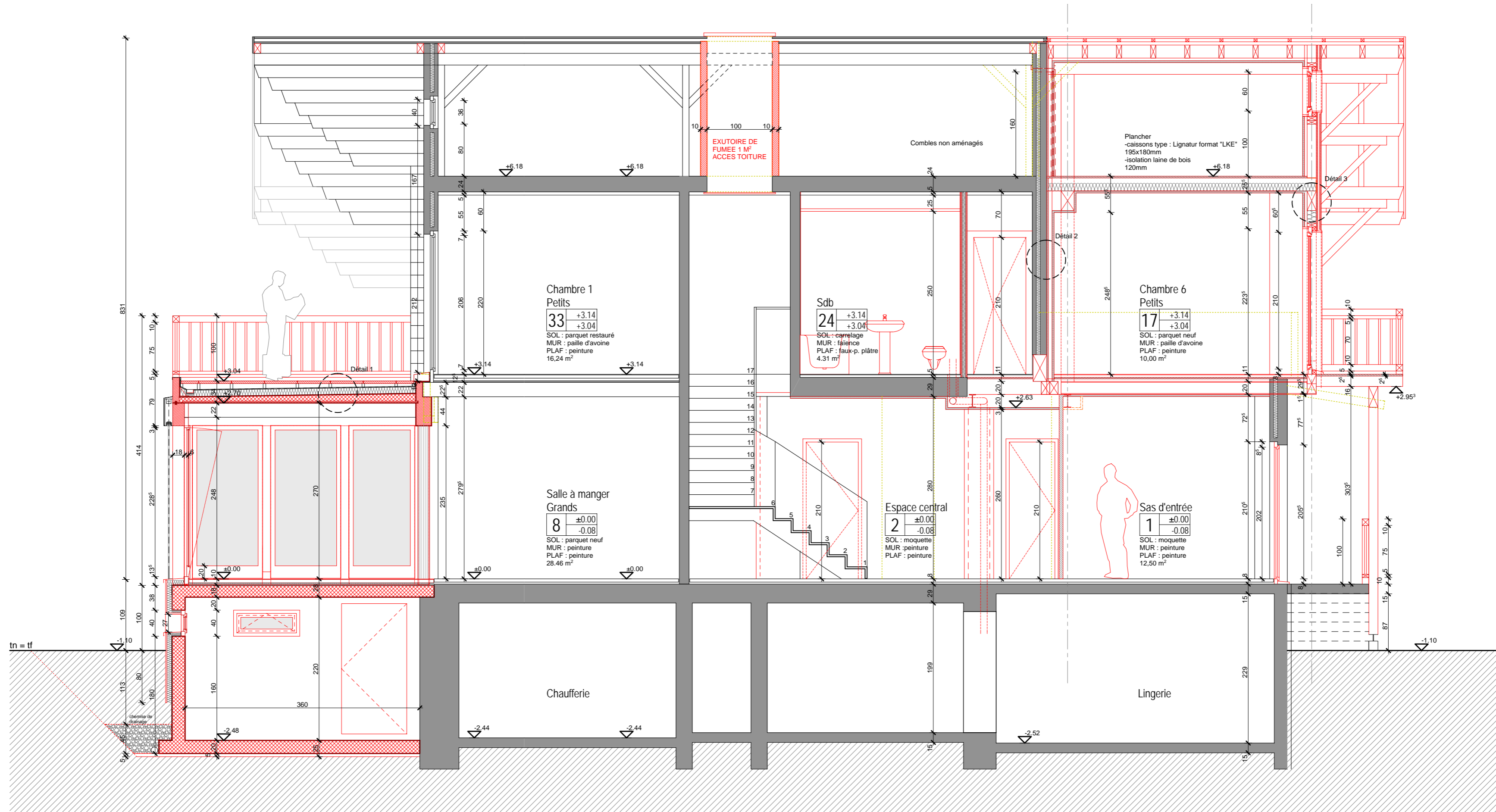
coupe A-A
