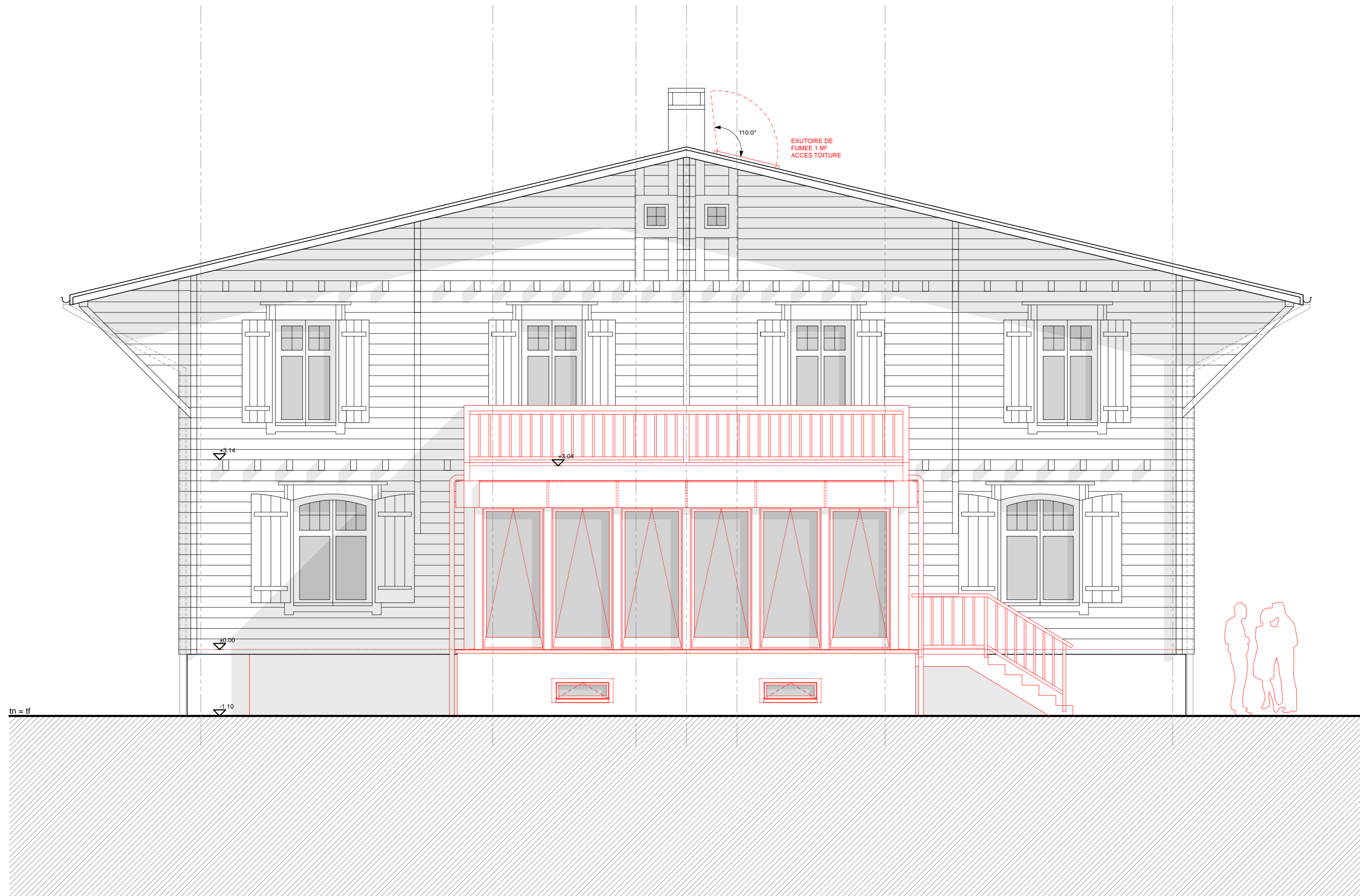
façade Sud-Ouest
