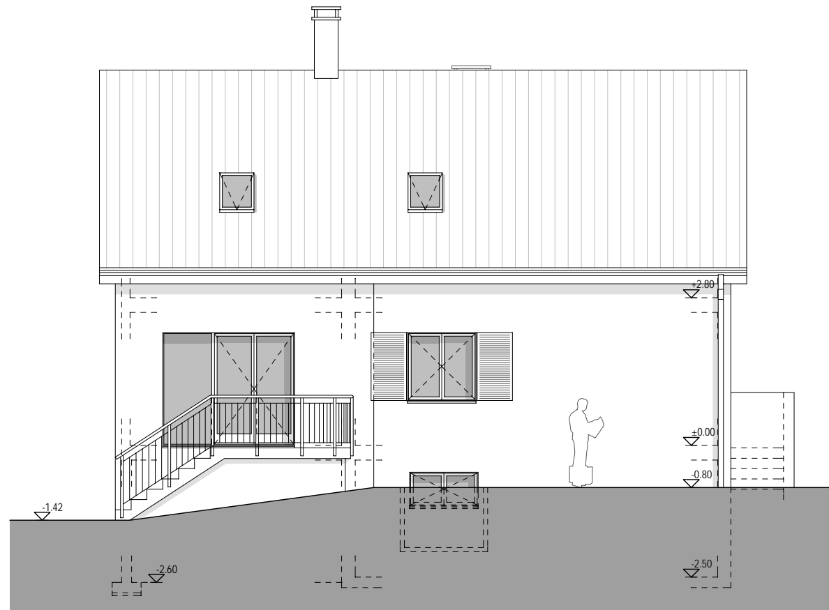
Façade Ouest
