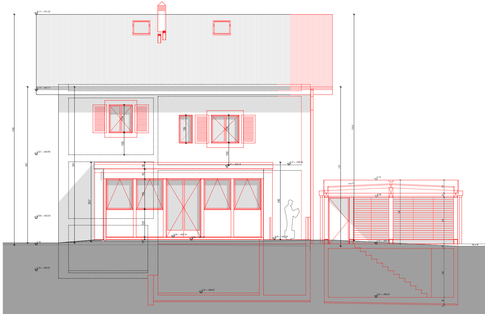
Façade nord-est
