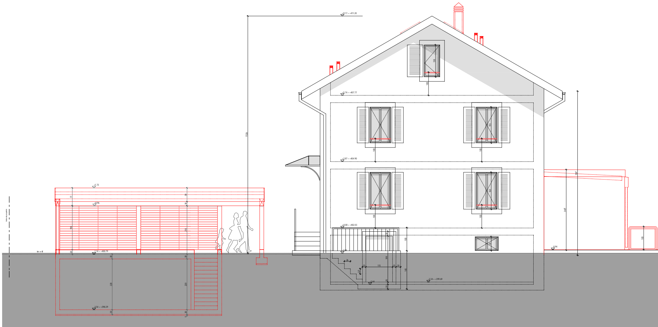
Façade sud-est
