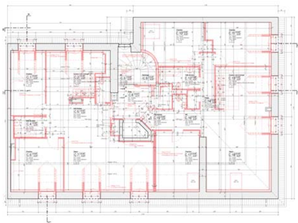
Plan des combles
